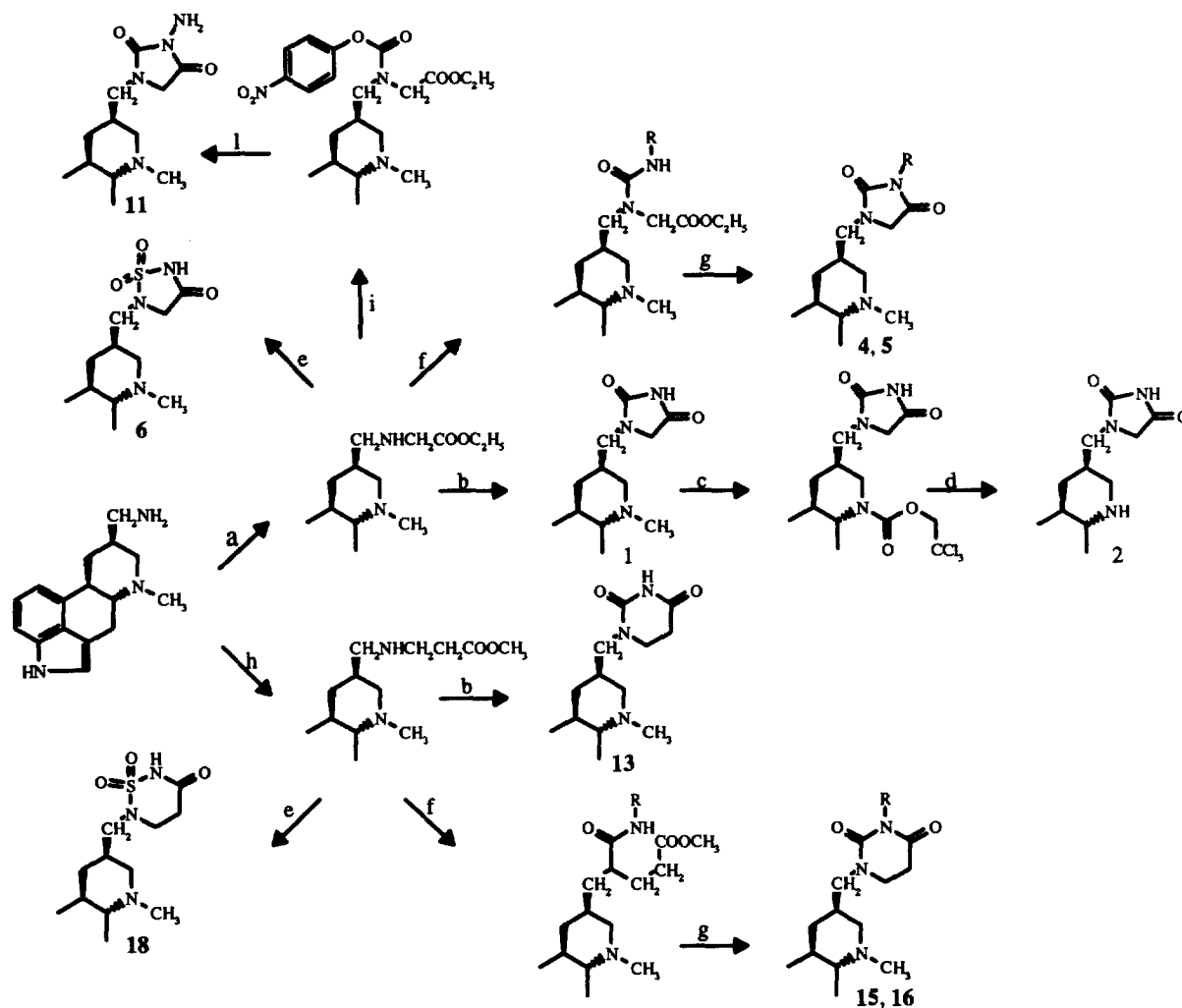
Fig. 3. (a) \text{BrCH}_2\text{COOC}_2\text{H}_5 , \text{K}_2\text{CO}_3 , DMF, r.t.; (b) \text{KOCN} , 1 N HCl, 90^\circ\text{C} ; (c) \text{CCl}_3\text{CH}_2\text{OCOC} , \text{KHCO}_3 , toluene, reflux; (d) powder Zn, AcOH, 35^\circ\text{C} ; (e) \text{NH}_2\text{SO}_2\text{NH}_2 , 150^\circ\text{C} ; (f) \text{RNCO} , dioxane, reflux; (g) 170^\circ\text{C} , vacuum; (h) \text{CH}_2=\text{CHCOOCH}_3 , dioxane, reflux; (i) p -nitrophenyl chlorocarbonate, pyridine, r.t.; (l) \text{NH}_2\text{NH}_2 , pyridine, reflux.
